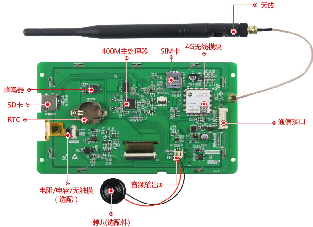
图 1-4 硬件配置图
